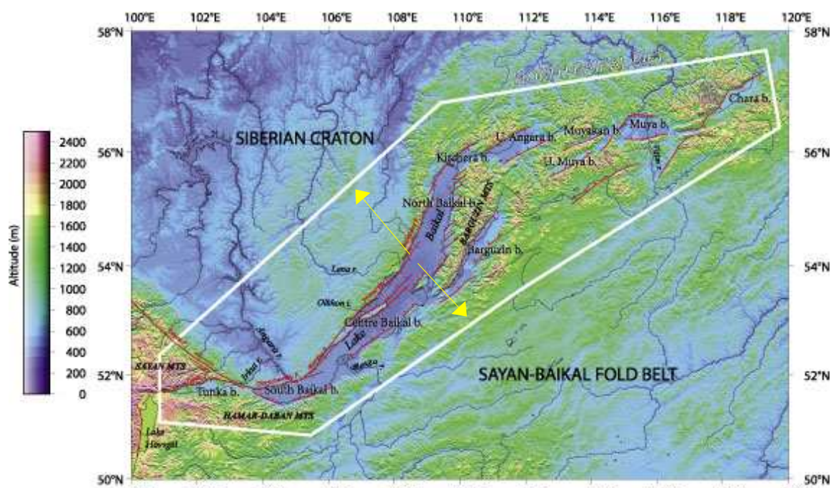
Figure 1 : représentation topographique du rift Baïkal. Flèches jaunes : direction moyenne d'extension.
