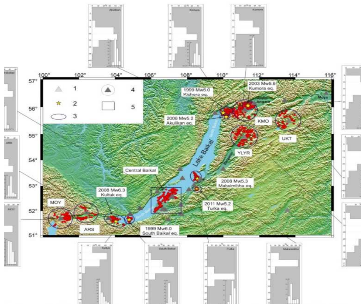
Figure 2 : Représentation du rift Baïkal et de quelques exemples de distributions en profondeur pour une ensemble de regroupements (clusters) sismiques identifiés en périodes intersismique ou post-sismique. L'année et la magnitude Mw des séismes suivis de répliques sont indiquées. Les codes des stations permanentes utilisées comme stations proches pour contraindre la profondeur des séismes sont indiquées pour les périodes intersismiques. Le rectangle représente une distribution intersismique au centre de Lac Baïkal. D'après A. Radziminovich (Pure Appl. Geophys., https://doi.org/10.1007/s00024-022-02952-x , 2022).
